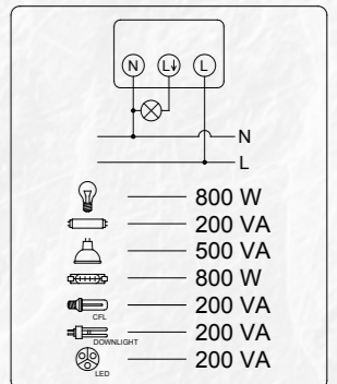
Caractéristiques techniques
