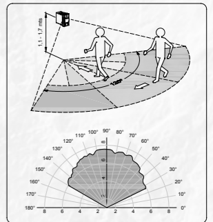
Caractéristiques techniques
